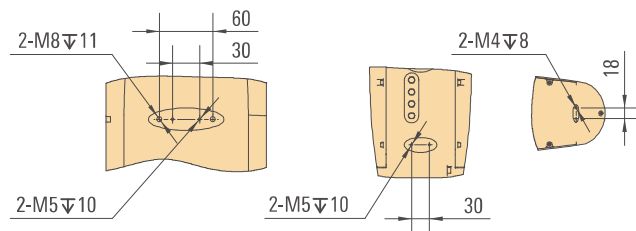
肘部孔位图 Elbow arm
