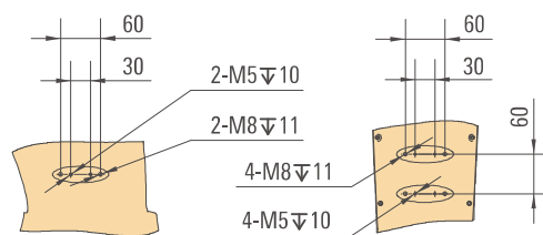
肩部孔位图 Shoulder arm
