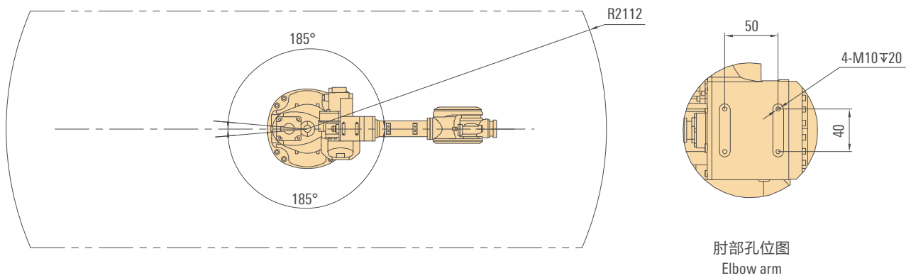
法兰图 Flange drawing
